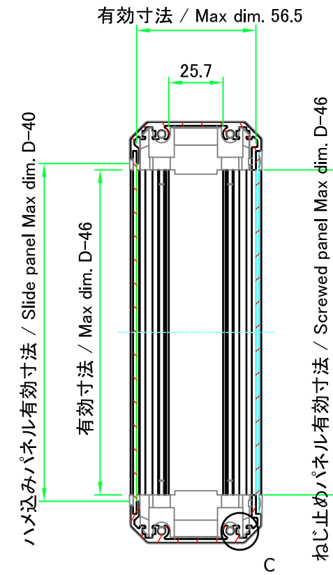
B-B ( 1 : 2.5 )
